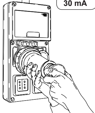
Conexión eléctrica.
