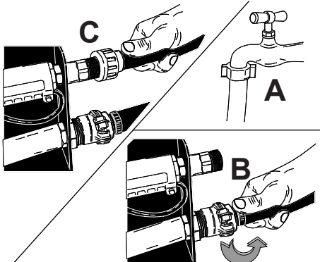
Collegamento idrico.
