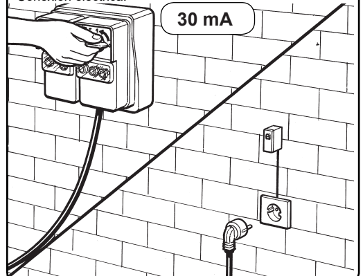
Conexión eléctrica.
